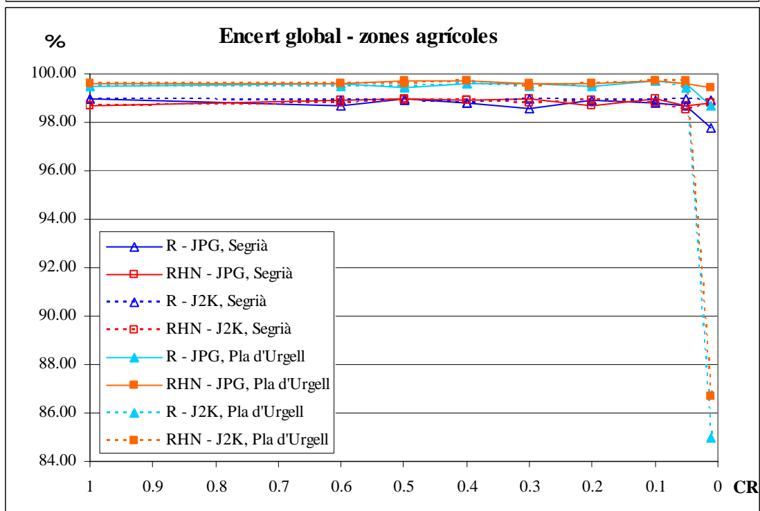
Figura 5: Resultats per a les zones agrícoles: Àrea cartografiada (gràfic superior) i Encert global (inferior) per la zona de la Segrià i Pla d'Urgell
